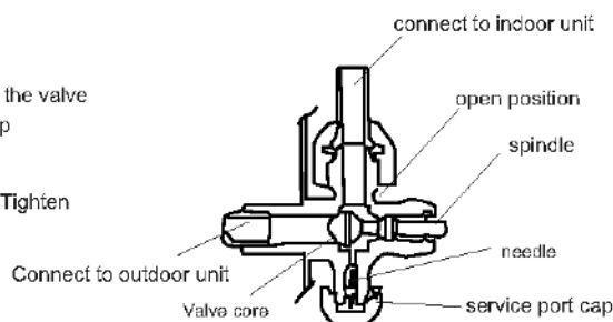
Esquema de la válvula de 3 vías
