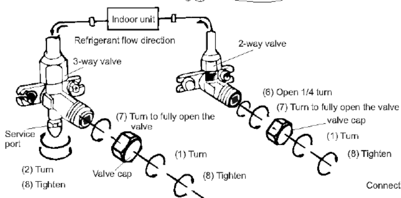
Schéma robinet à trois voies
