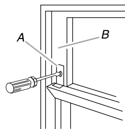
A. Patte de blocage de la fenêtre B. Fenêtre supérieure
