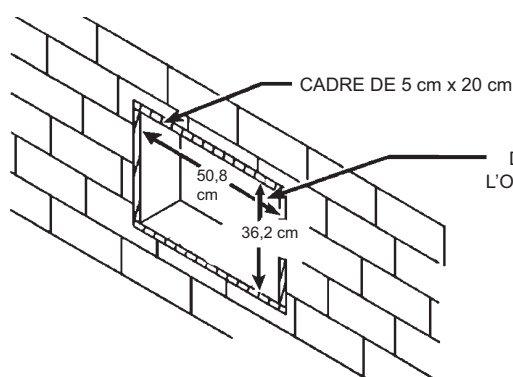
CONSTRUCTION À BLOCS EN BÉTON
