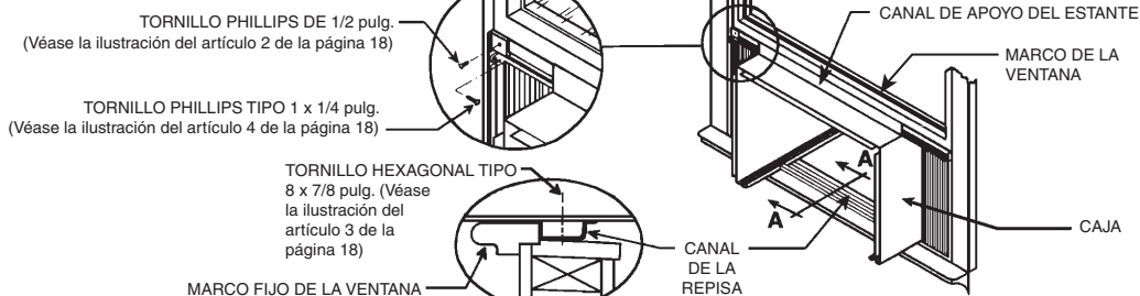
SECCIÓN A-A
