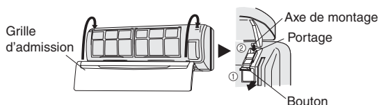
Grille d'admission
