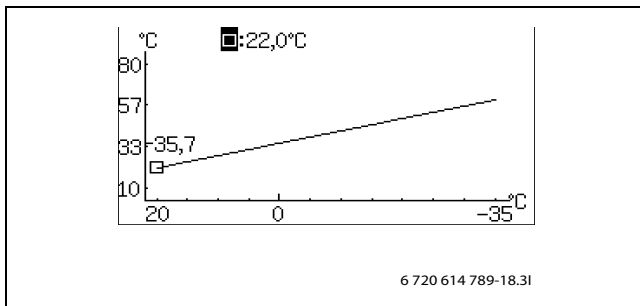
Fig. 22 Indstillingsvinduet Varmekurve (radiator)
