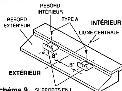
Schéma 9 SUPPORTS EN L
