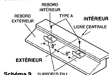
Schéma 9 SUPPORTS EN L
