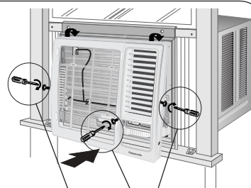
Chassis locking brackets Soportes que cierran el chasis
